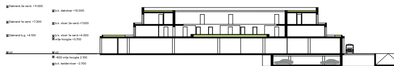
Doorsnede D
