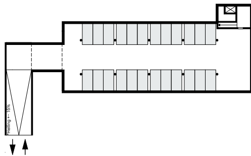
-1. Schematische weergave Stallingsgarage onder supermarkt 2
