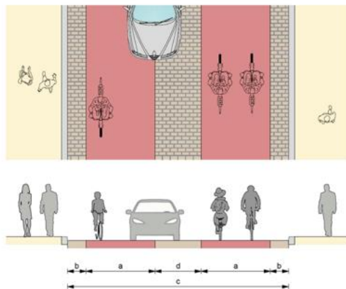
Fietsstraat breed profiel (4,5-7,3 m)
