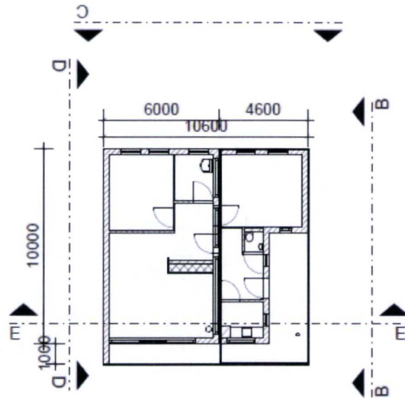
Grondplan
