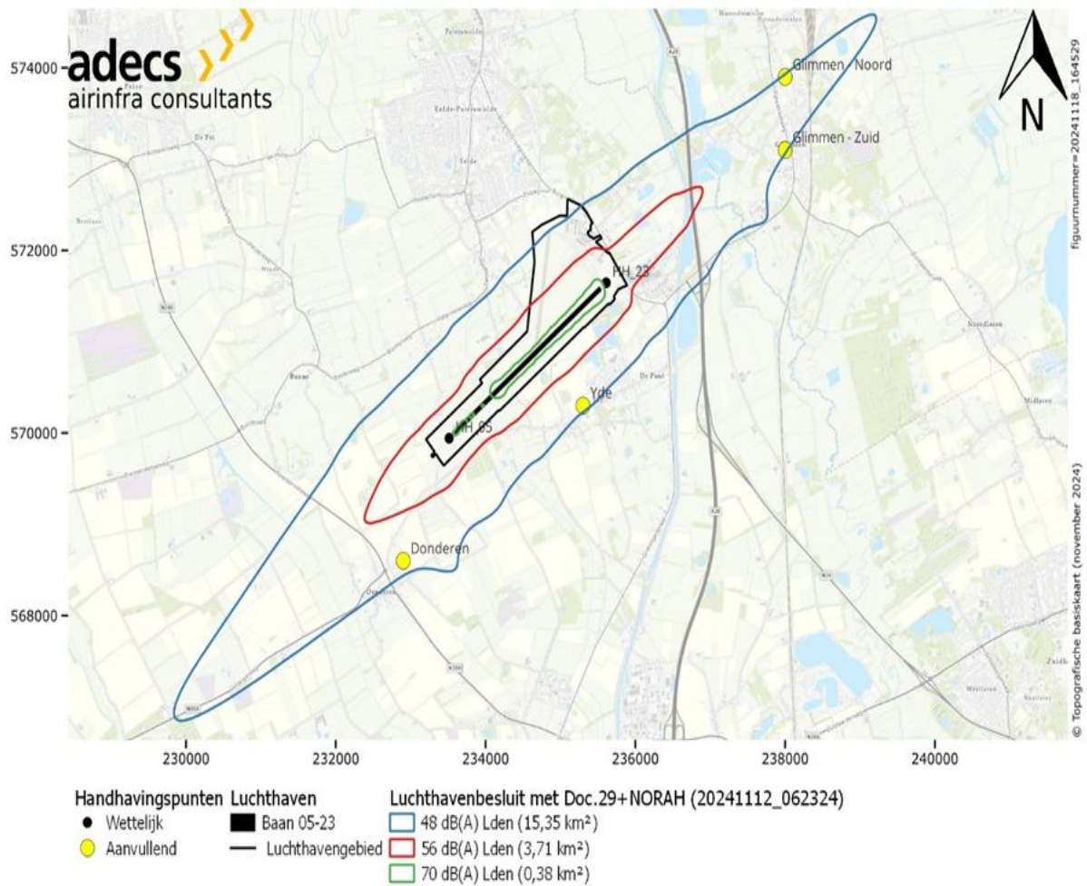
Figuur 1 Advies locatie handhavingspunten en ligging 48, 56 en 70 dB(A) Lden-contouren voor luchthaven Eelde.
